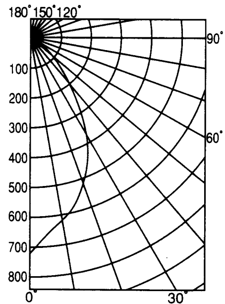
配光曲线
